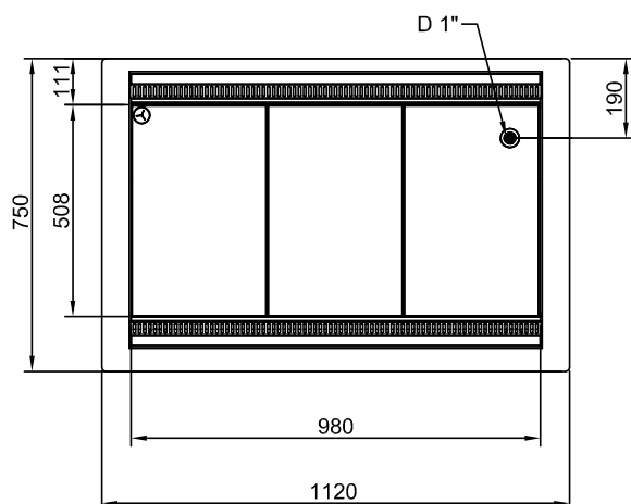
Boven aanzicht
